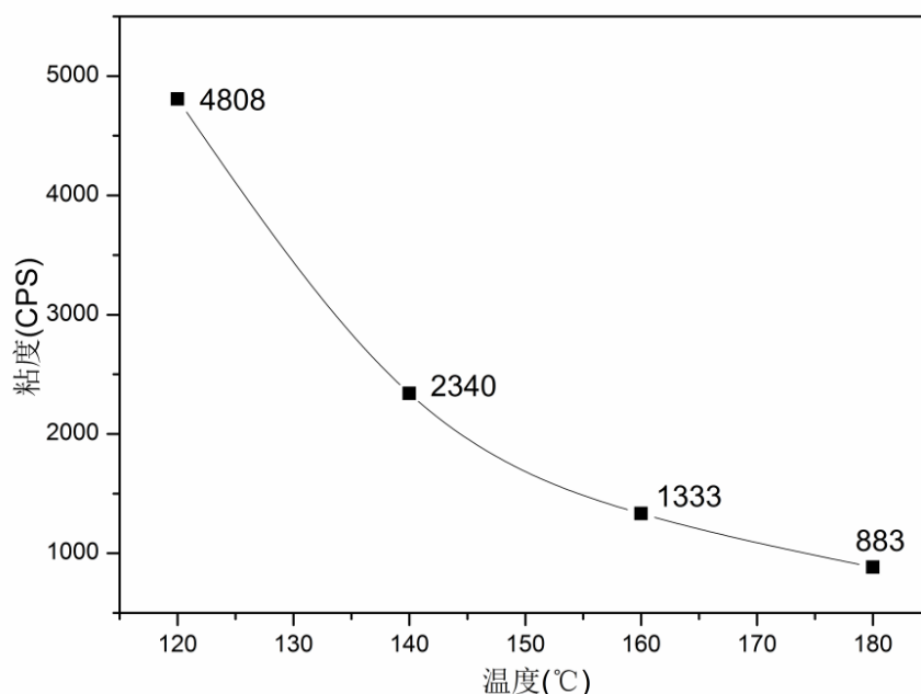
图1、EVA封箱胶粘度随温度变化图
